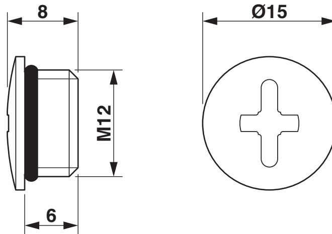
Disegno quotato
