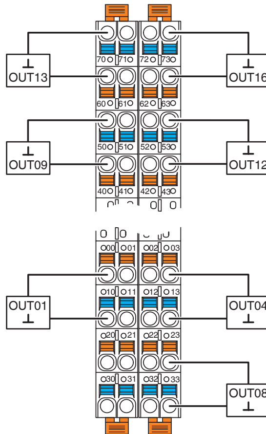
Disegno collegamento
