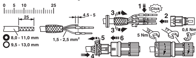
Disegno funzionamento
