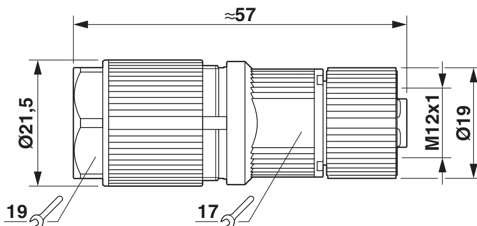
Disegno quotato
