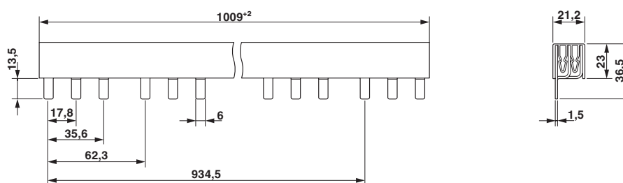
Disegno quotato
