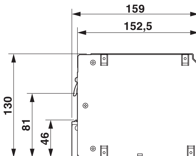
Disegno quotato
