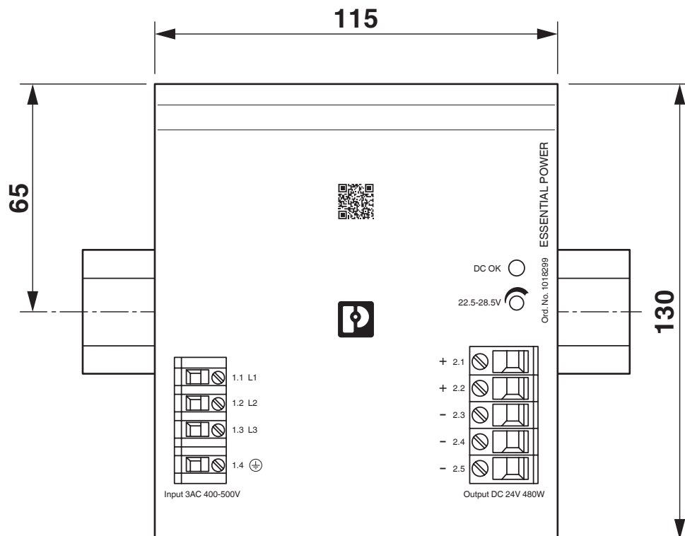
Disegno quotato
