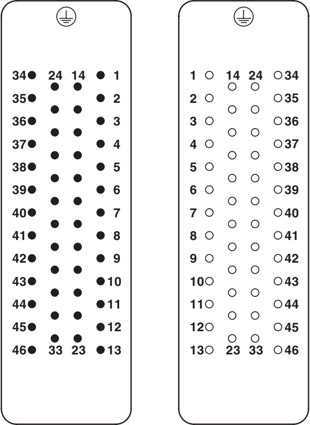
Disegno schema
