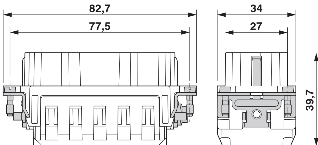
Inserto portacontatti femmina
