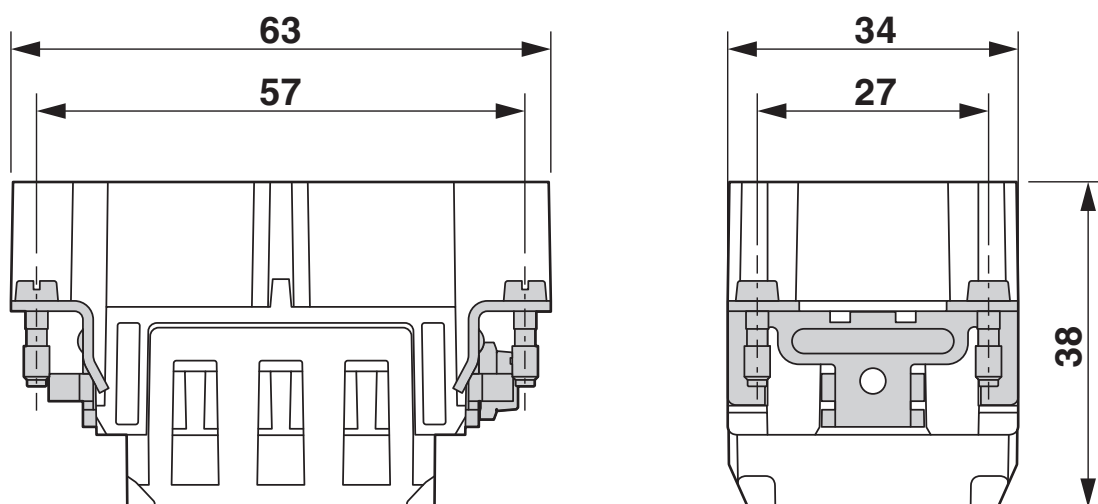
Inserto portacontatti maschio
