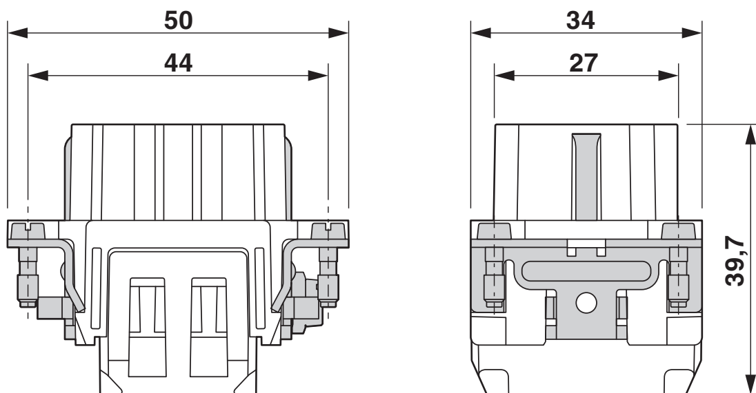
Inserto portacontatti femmina
