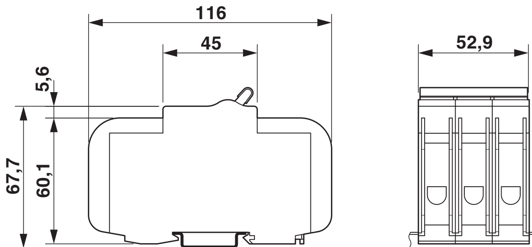
Disegno quotato
