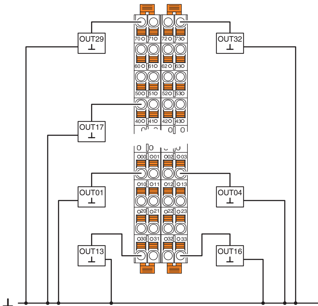
Disegno collegamento
