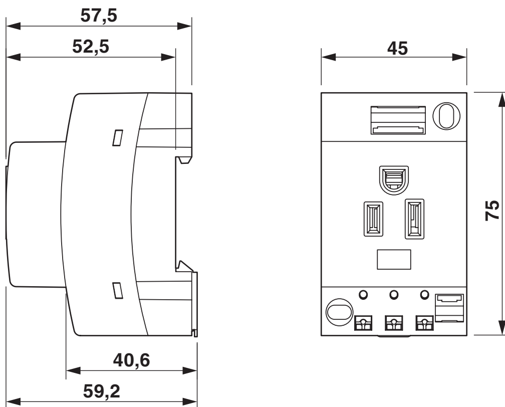
Disegno quotato
