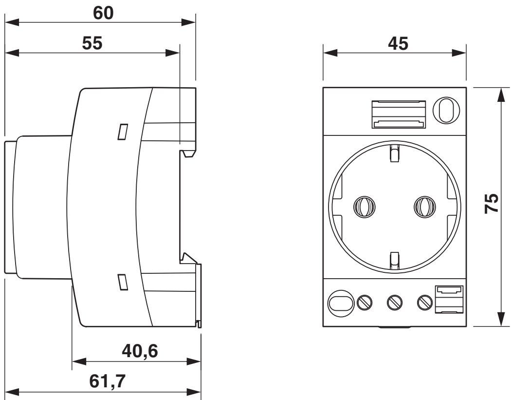
Disegno quotato
