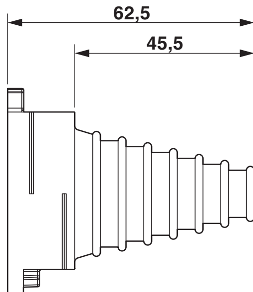
Disegno quotato
