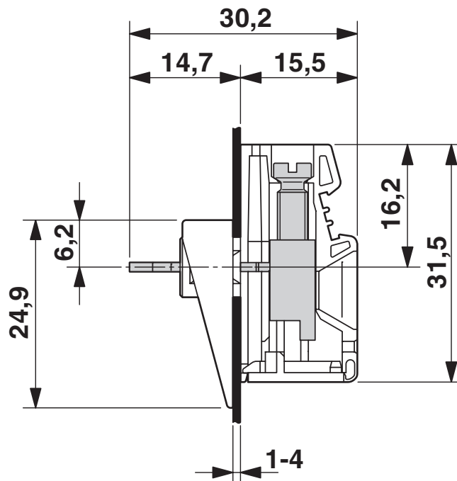
Disegno quotato
