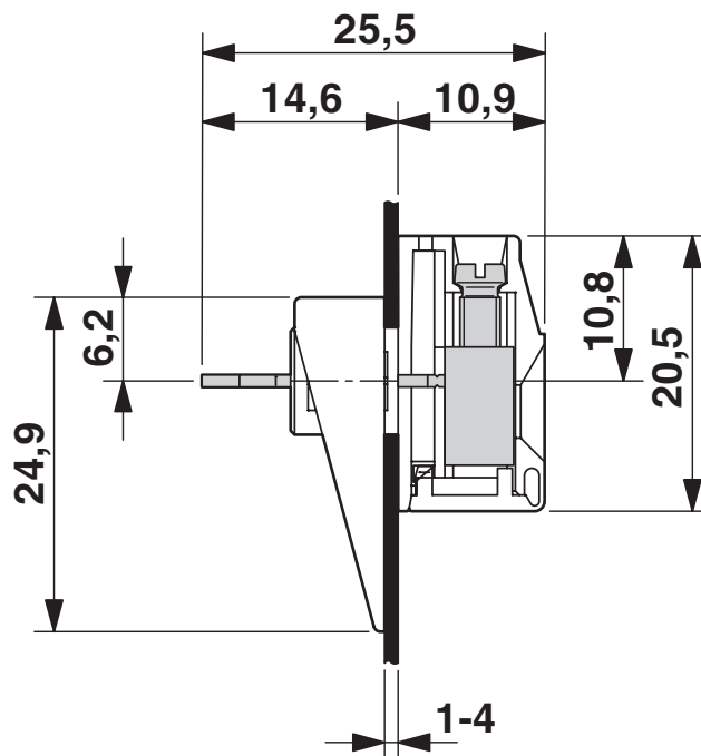
Disegno quotato
