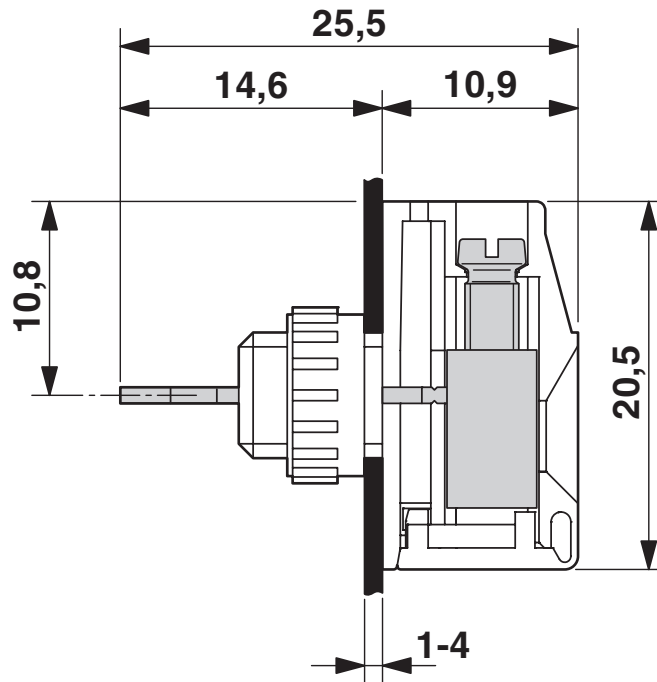
Disegno quotato
