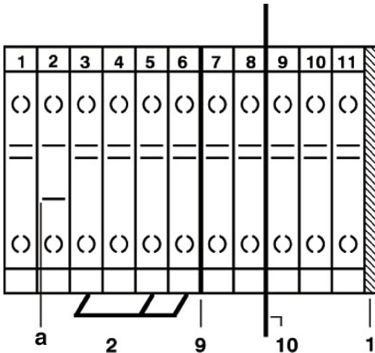
Schema di collegamento
