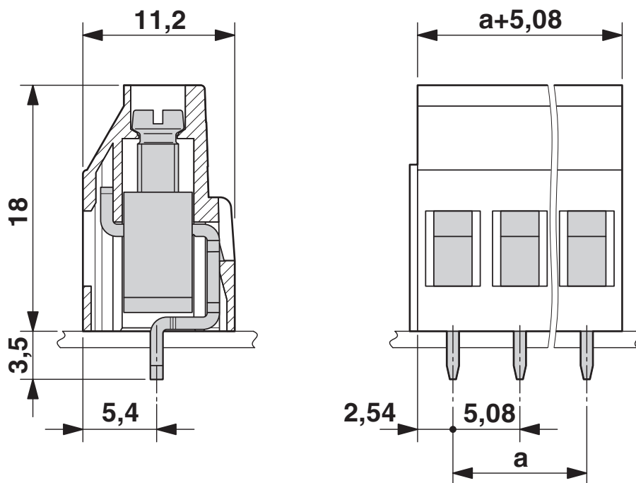
Disegno quotato
