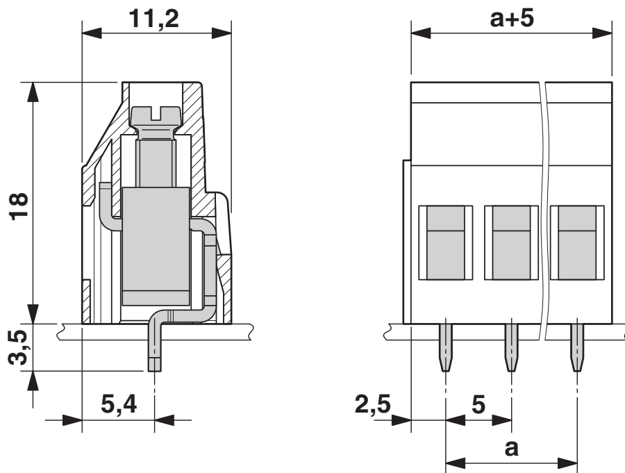
Disegno quotato
