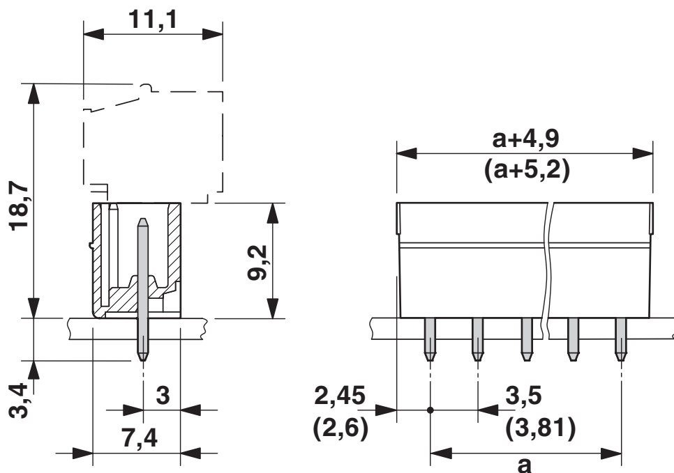
Disegno quotato
