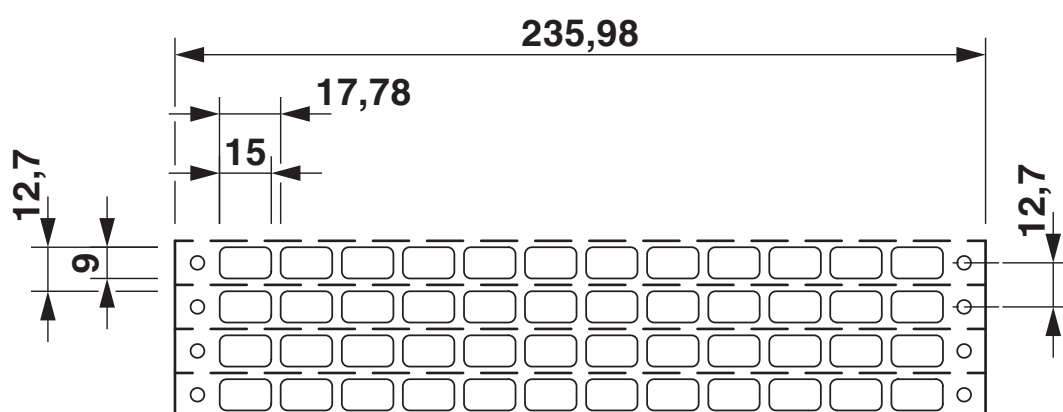
Disegno quotato
