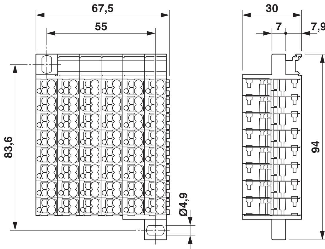
Disegno quotato
