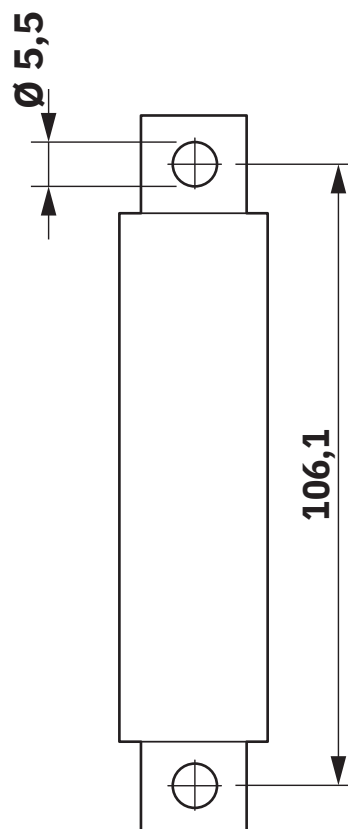
Disegno quotato
