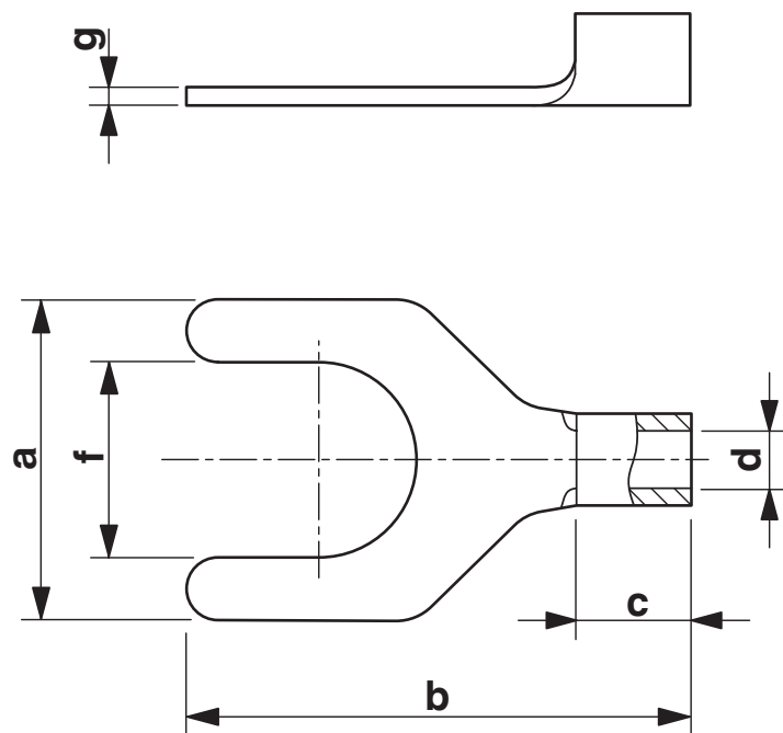
Disegno quotato
