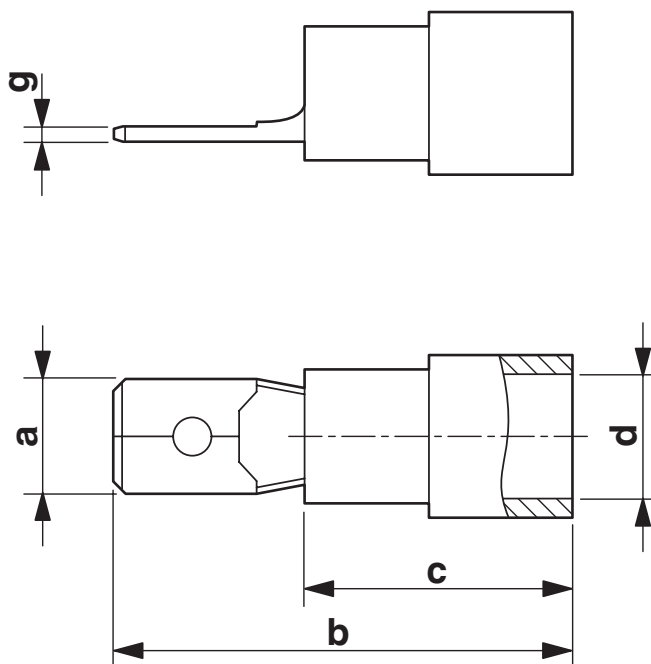
Disegno quotato
