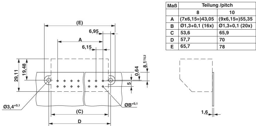
Disegno quotato
