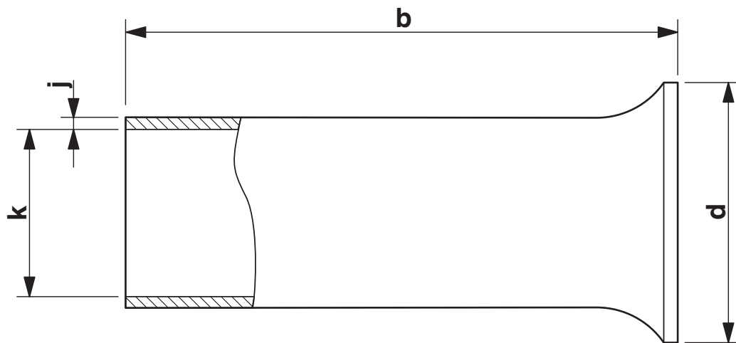
Disegno quotato
