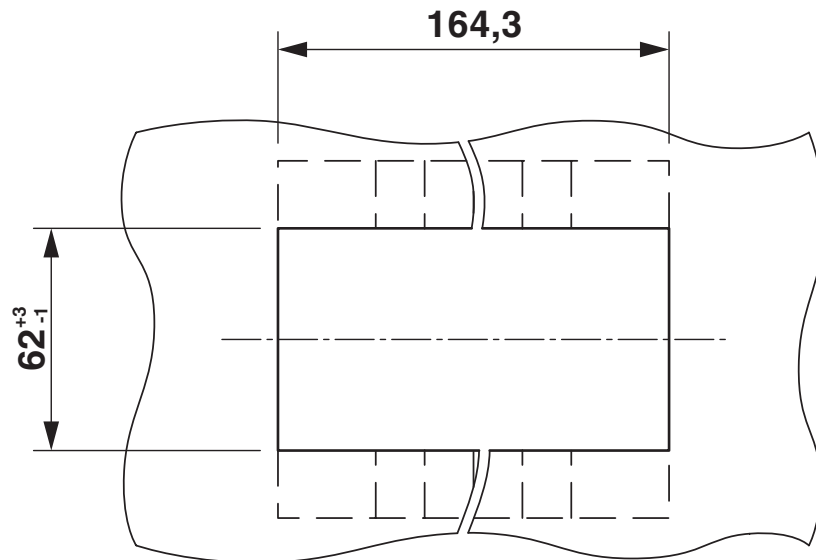
Disegno quotato
