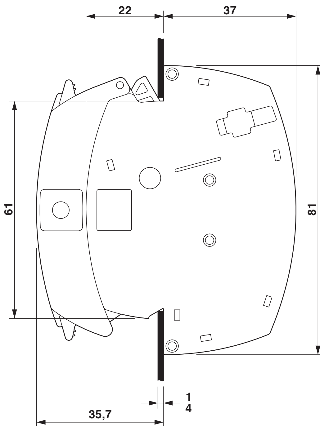
Disegno quotato
