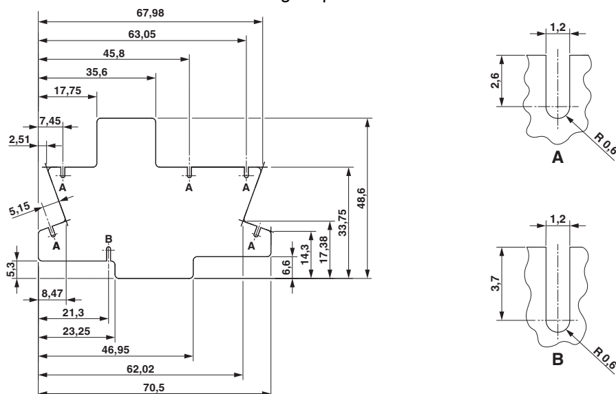
Disegno quotato delle asole del c.s. (particolare A e B) metallizzate nella zona aperta
