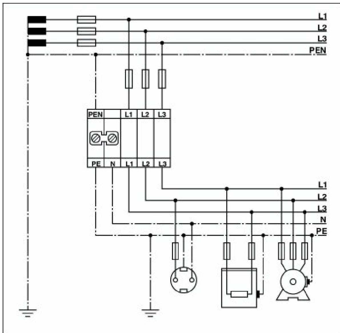
Disegno collegamento
