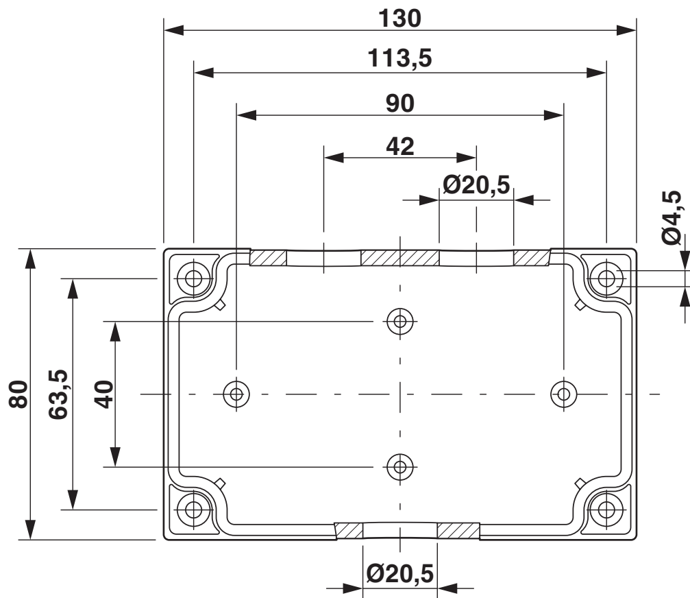
Disegno quotato
