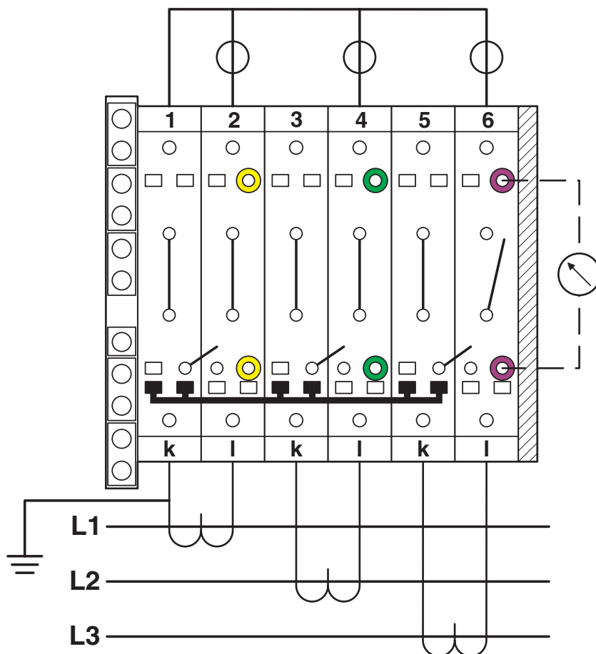
Disegno collegamento
