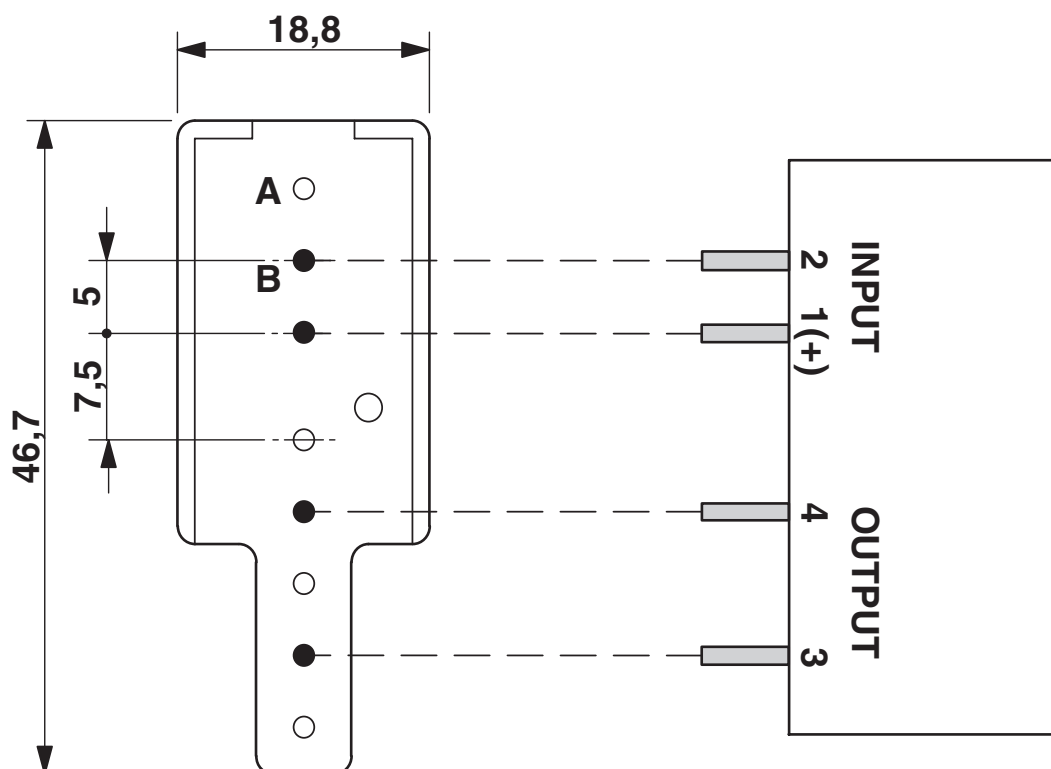
Disegno quotato
