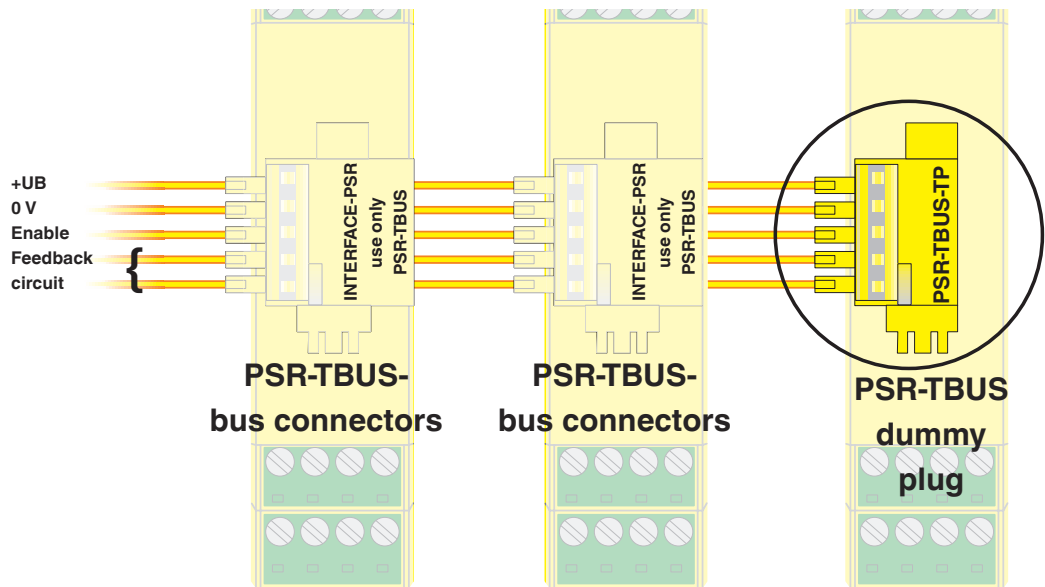
Disegno collegamento
