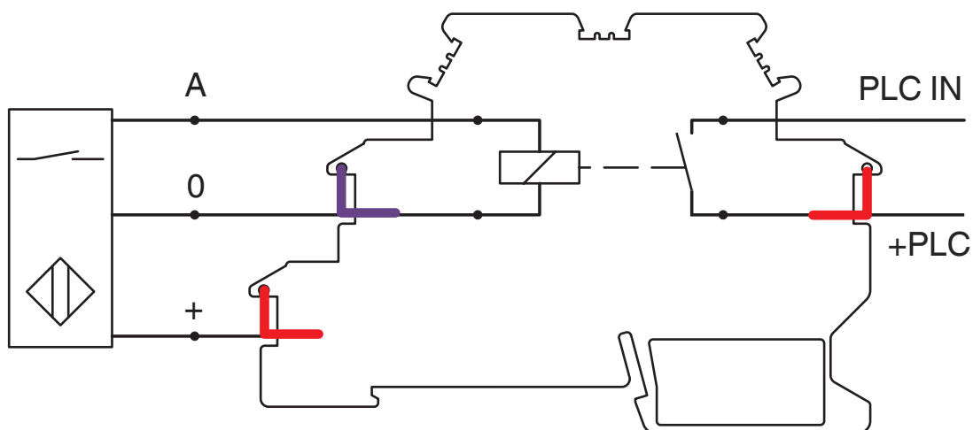
Piedinatura DEK-REL-...SEN
