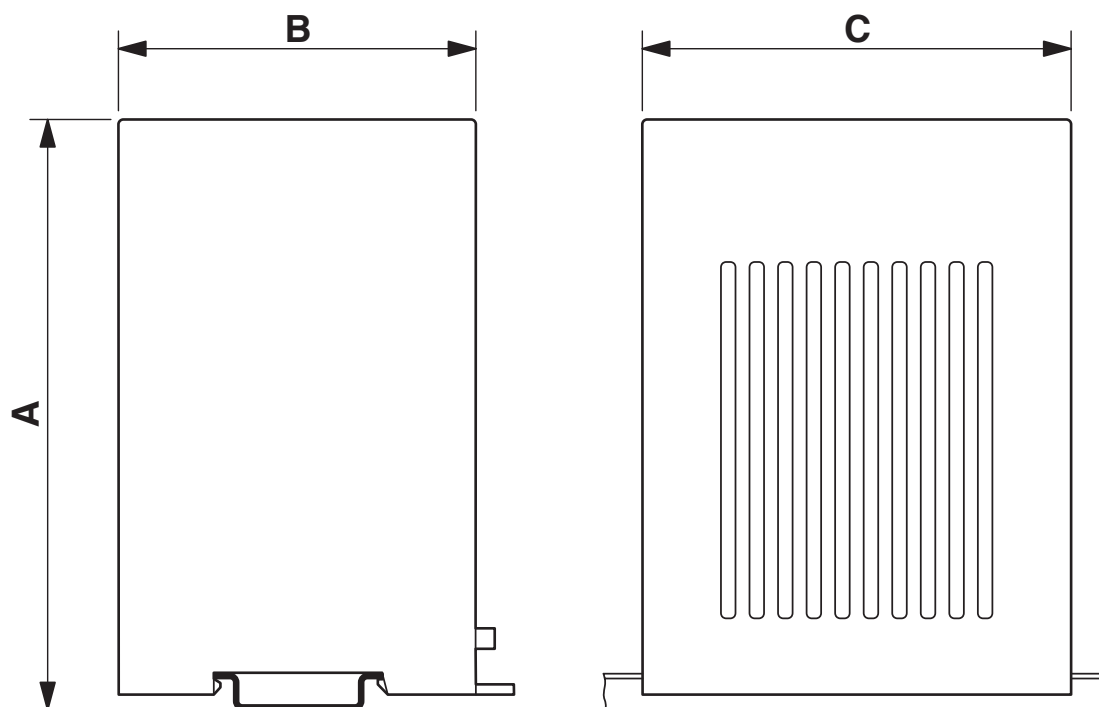
Disegno quotato
