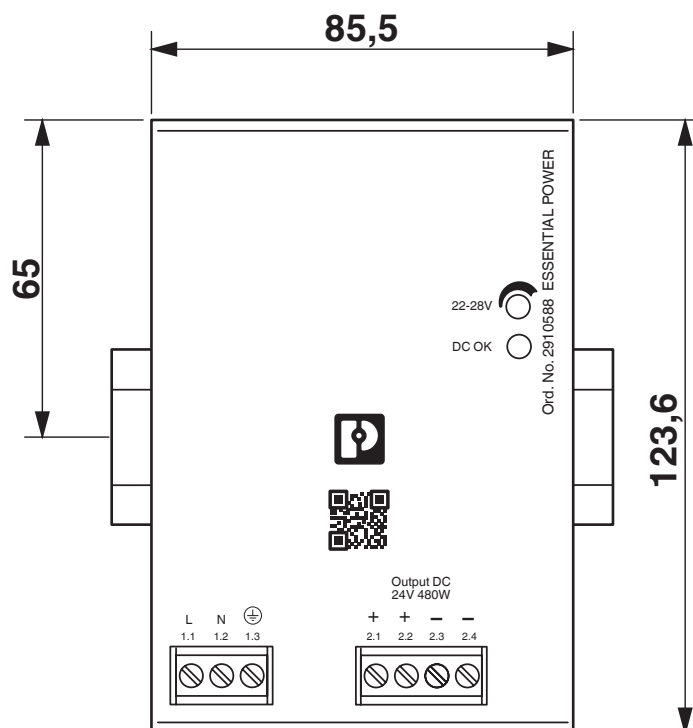
Disegno quotato
