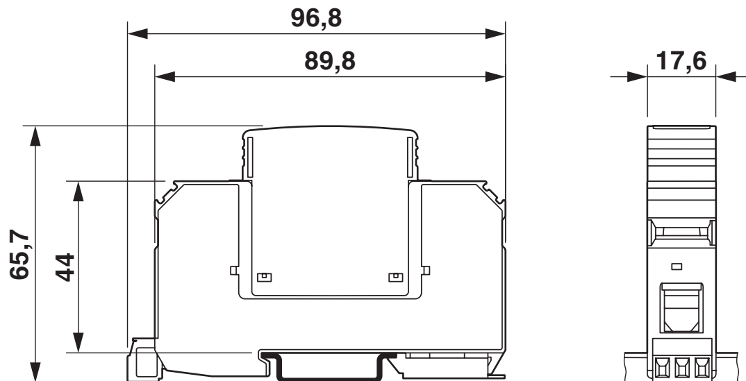
Disegno quotato
