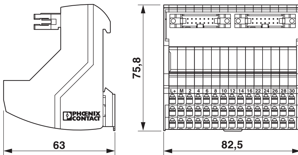
Disegno quotato
