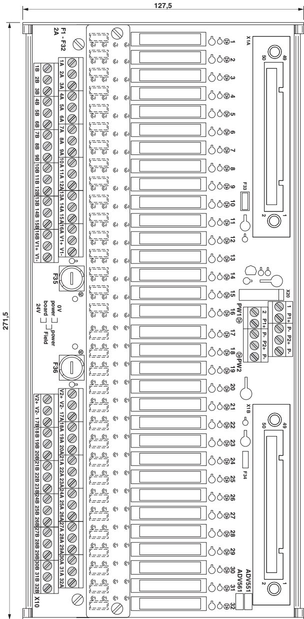
Disegno quotato
