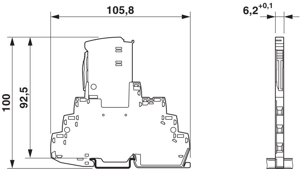
Disegno schema
