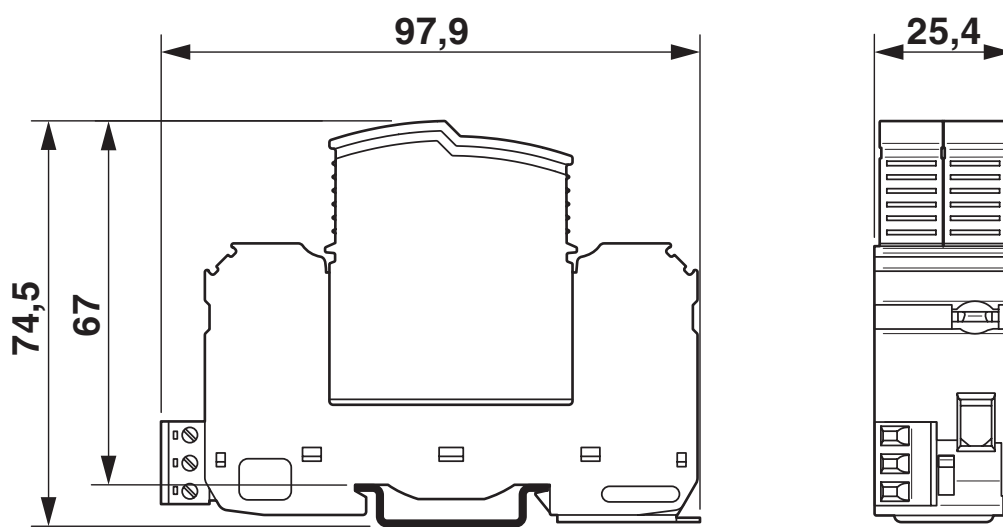
Disegno quotato
