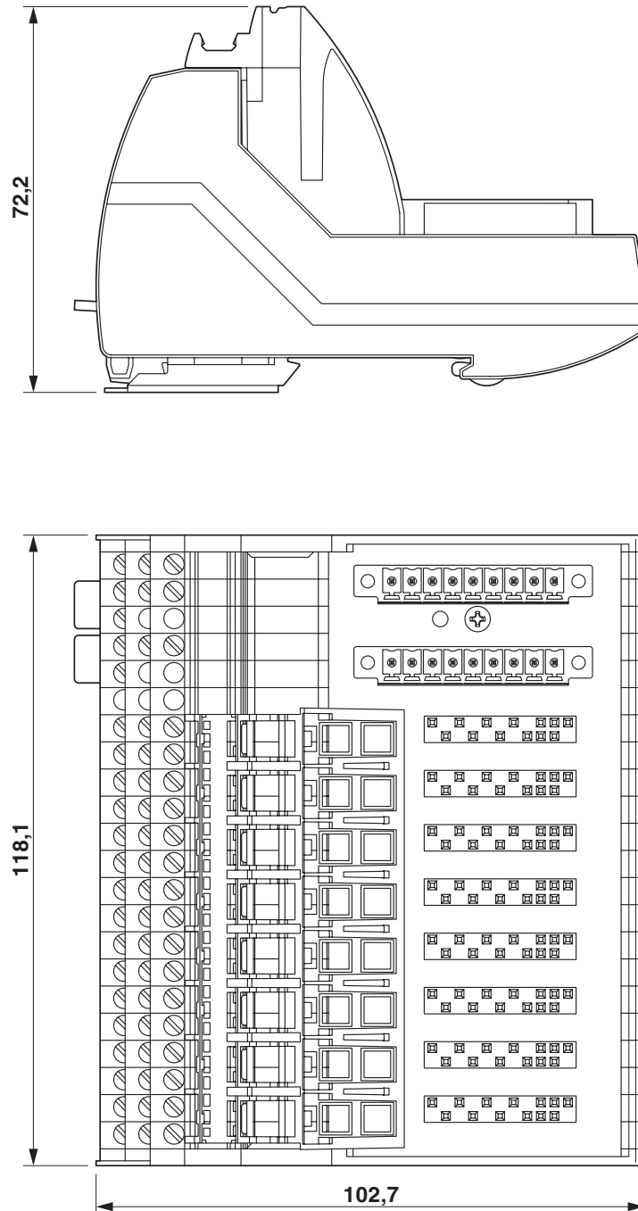
Disegno quotato
