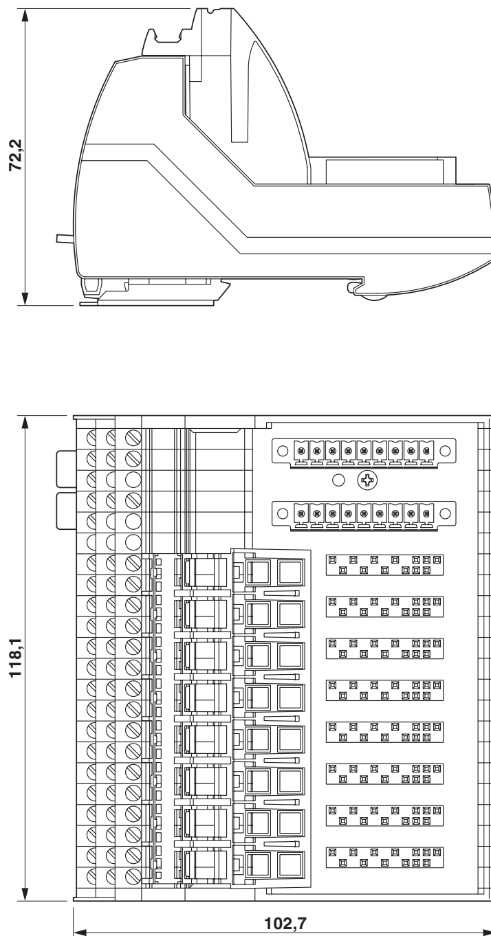
Disegno quotato
