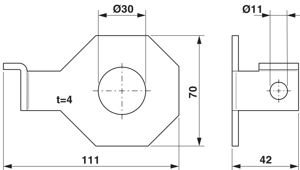
Disegno quotato
