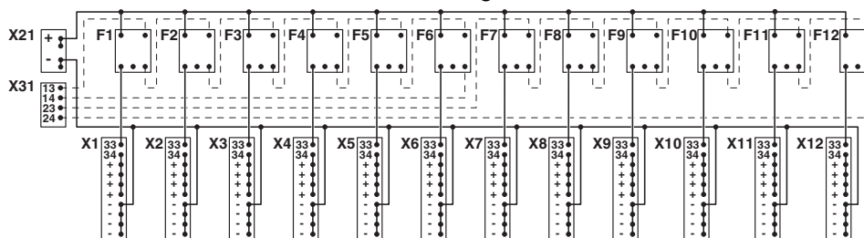
Schema di collegamento
