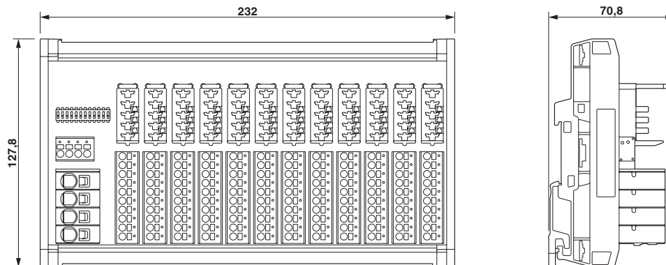
Disegno quotato
