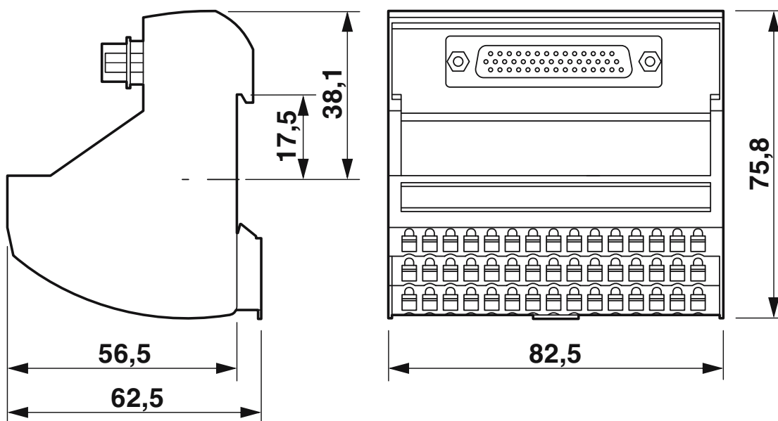
Disegno quotato
