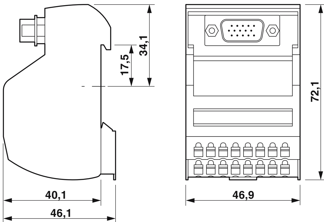
Disegno quotato
